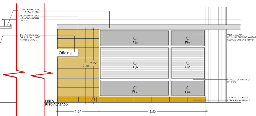
FACHADA TIPO B
