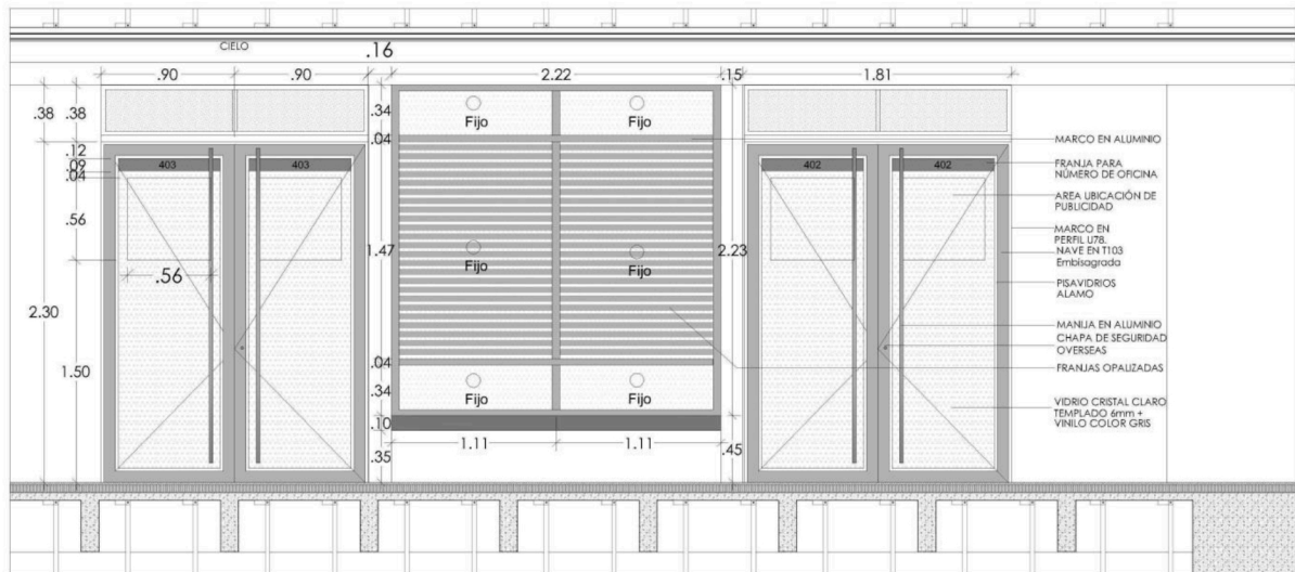
SECCIÓN TIPO OFICINAS
