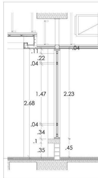
SECCIÓN TIPO OFICINAS
