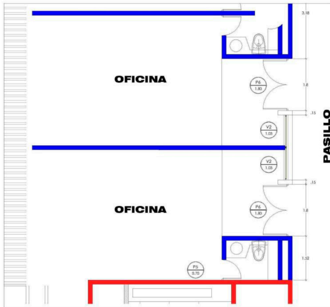
PLANTA TIPO OFICINAS
